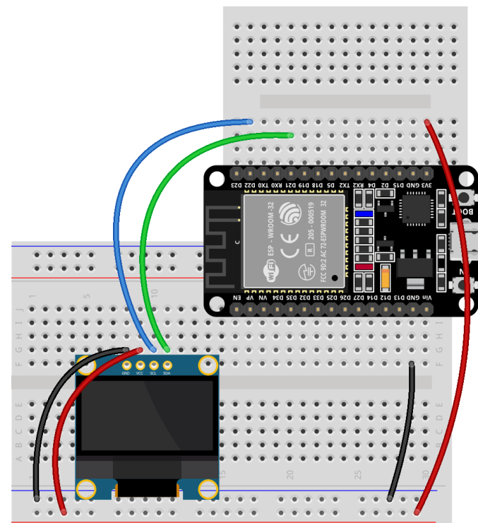
Рисунок 7. SSD1306
