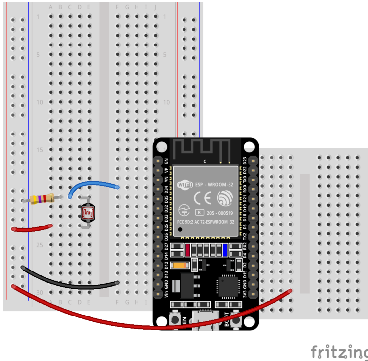
Рисунок 4. Фоторезистор
