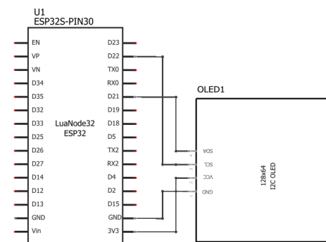
Рисунок 8. SSD1306
