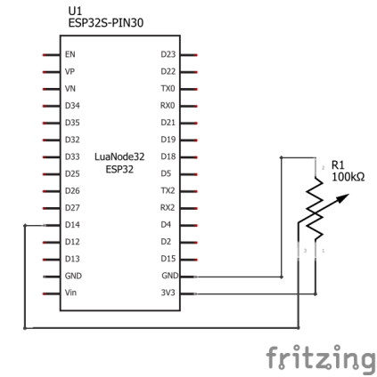
Рисунок 3. Потенциометр
