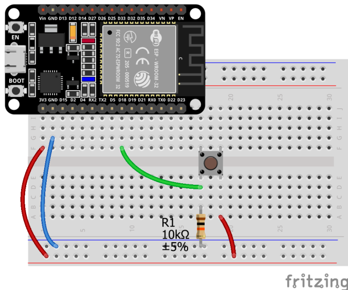
Рисунок 1. Кнопка
