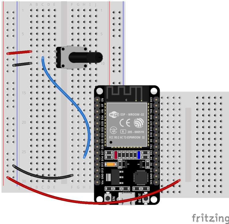
Рисунок 2. Потенциометр
