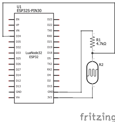
Рисунок 5. Фоторезистор
