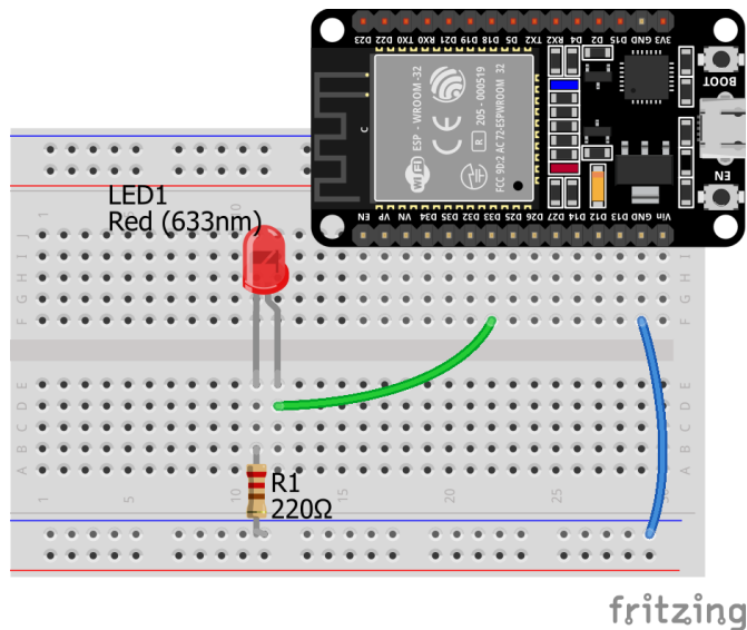
Рисунок 6. Светодиод
